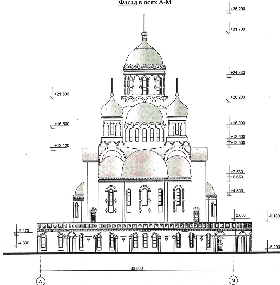
Фасад в осях А-М
