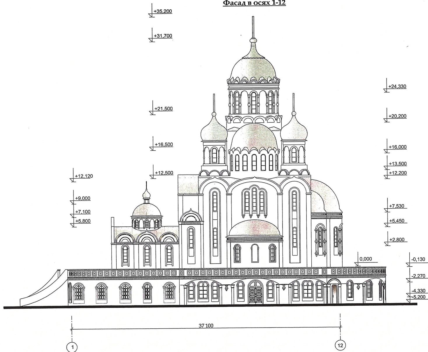
Фасад в осях 1-12
