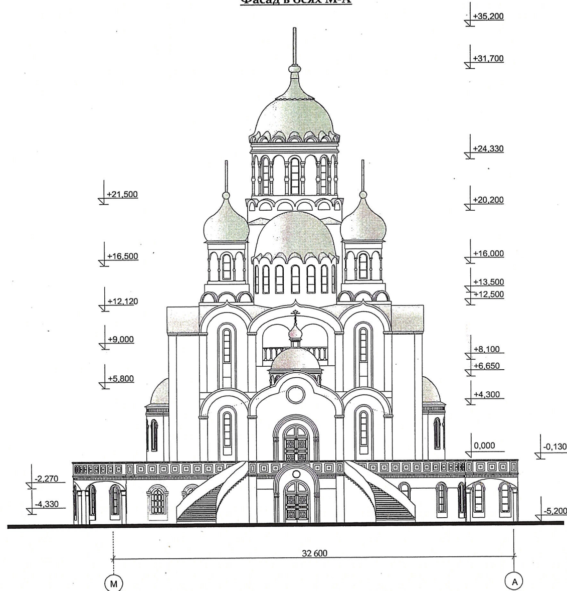
Фасад в осях М-А
