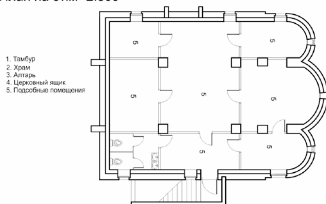
План на отм. -2.800
