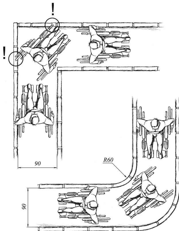
Рис. 2 Закругление путей движения (в см)
