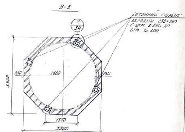
Схема монолитного пояса на отм.12.600
