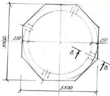
Схема монолитного пояса на отм.12.600
