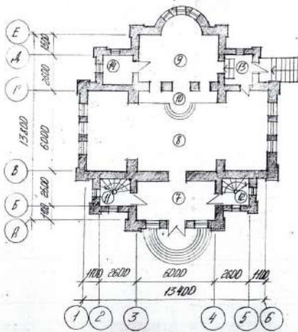
ПЛАН НА ДТМ 0.000
