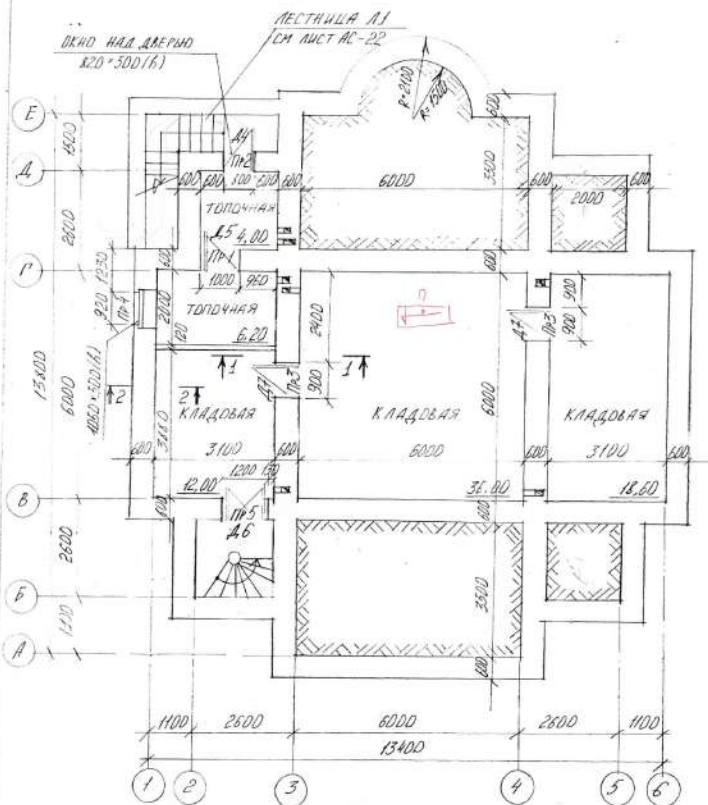
ПЛАН НА ДТМ. -3.450 М 1:100
