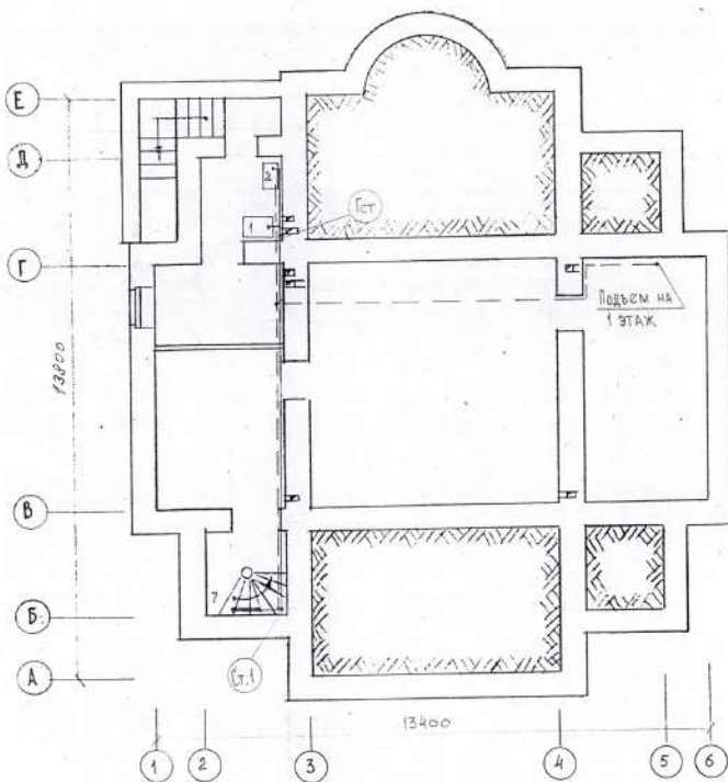
ПЛАН НА ОТМЕТКЕ -3,45 м
