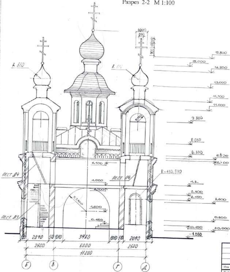
Разрез 2-2 М 1:100
