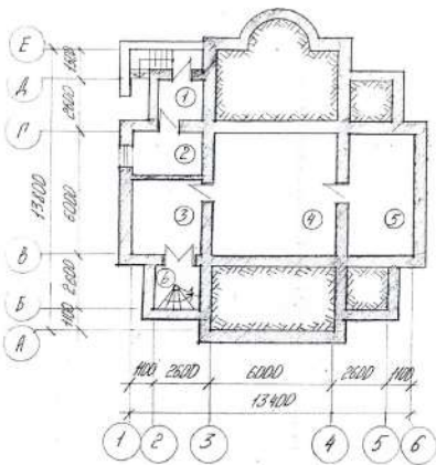
ПЛАН НА ДТМ 0.000
